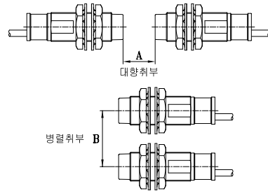
상호간 취부그림
