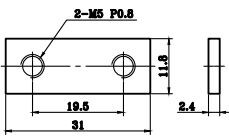
KH-6045
