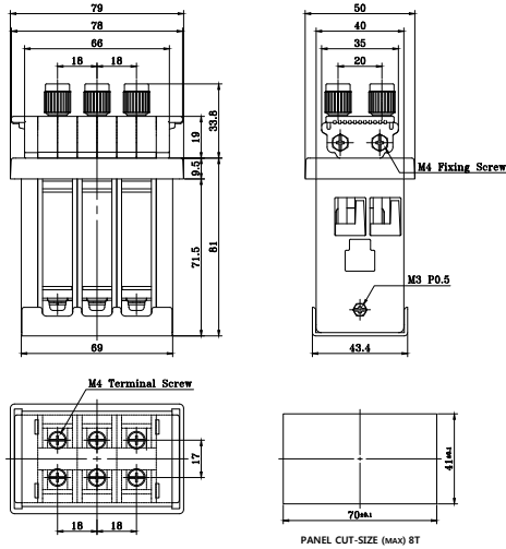
KTS-P, C-3P
