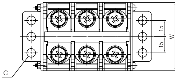
면취부형
