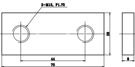
KH-60300, KH-60400
