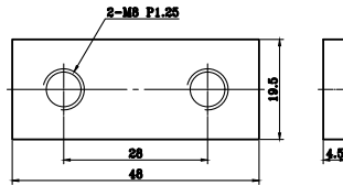
KH-60100
