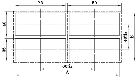
패널가공방법 A(mm)=80×열수-5 B(mm)=40×단수-5
