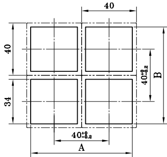
패널가공방법 A(mm)=40×열수-5 B(mm)=40×단수-5
